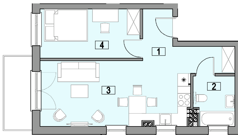
PLAN MIESZKANIA 1:100
