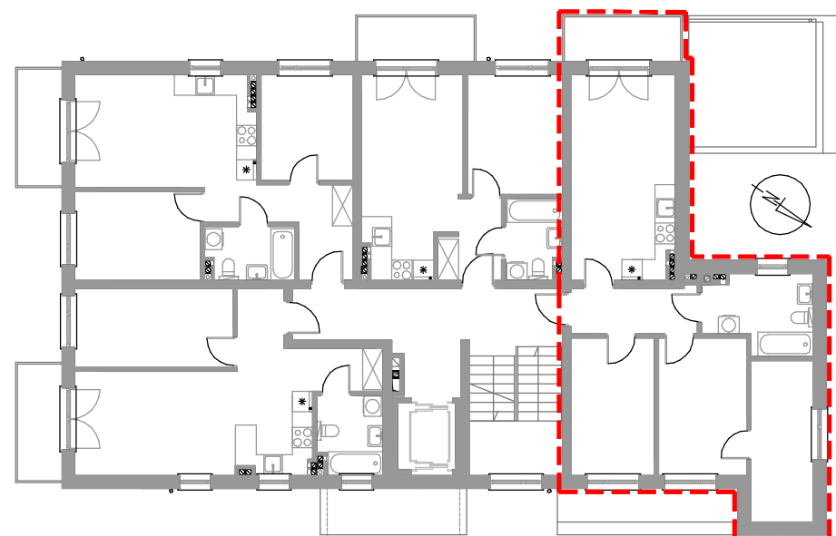
RZUT KONDYGNACJI Z OZNACZENIEM LOKALU
