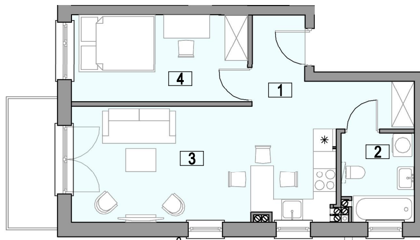
PLAN MIESZKANIA 1:100
