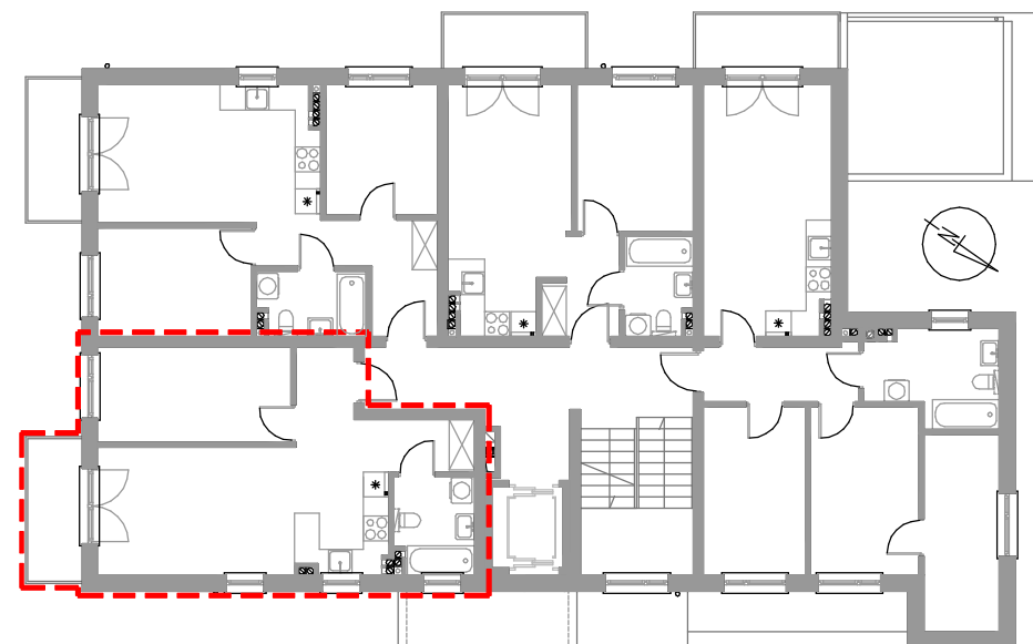
RZUT KONDYGNACJI Z OZNACZENIEM LOKALU
