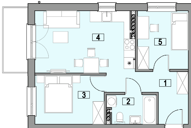
PLAN MIESZKANIA 1:100
